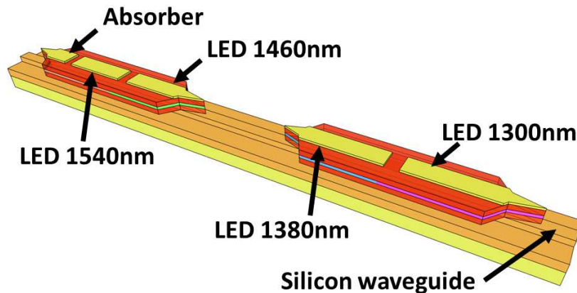
Figuur 3: Illustratie van een SLED op SOI bestaande uit 4 actieve bandkloven, gecreëerd door middel van QWI en multiple die bonding
